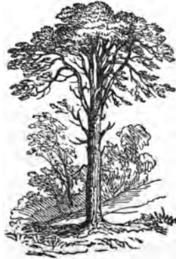
PINUS SYLVESTUS. (Scotch Fir.)
